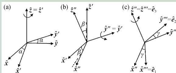
图3 欧拉角 \alpha, \beta, \gamma 的定义。从实验室坐标系 (\hat{x}, \hat{y}, \hat{z}) 出发绕着 \hat{z} 轴旋转 \alpha ，得到坐标系 (\hat{x}', \hat{y}', \hat{z}' = \hat{z}) 。再绕着 \hat{y}' 轴旋转 \beta ，得到坐标系 (\hat{x}'', \hat{y}' = \hat{y}', \hat{z}'') 。再绕着 \hat{z}'' 轴旋转 \gamma ，得到本体坐标系 (\hat{e}_1, \hat{e}_2, \hat{e}_3 = \hat{z}''')
