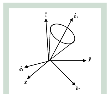
图2 实验室坐标系 (\hat{x}, \hat{y}, \hat{z}) 和固定在陀螺上的随动本体坐标系 (\hat{e}_1, \hat{e}_2, \hat{e}_3) 。它们之间由一个三维正交转动矩阵 \mathbf{g}(\alpha, \beta, \gamma) 相联系，其中 \alpha, \beta, \gamma 是欧拉角
